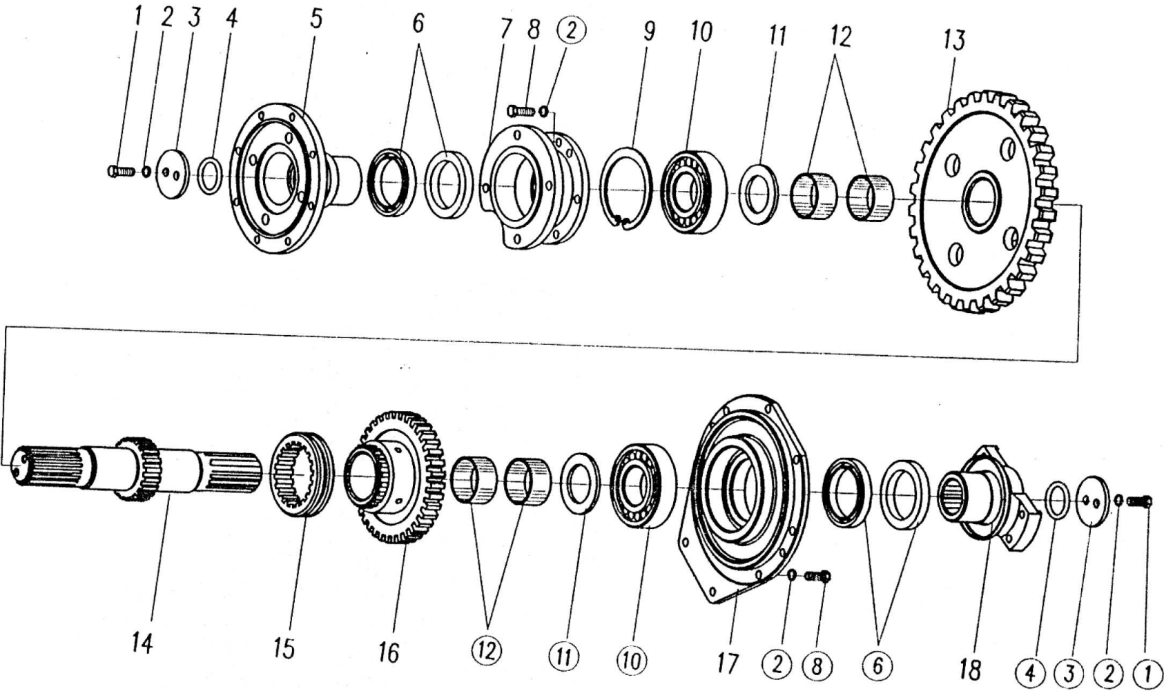
输出轴总成 Output shift assembly
